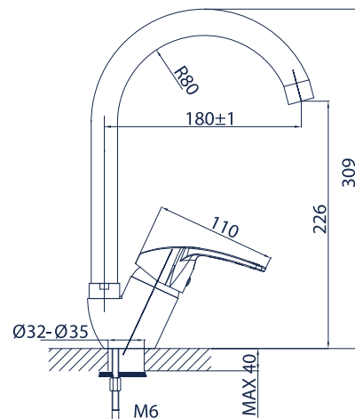
bateria zlewozmywakowa rurowa
