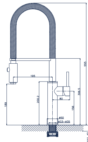
bateria zlewozmywakowa OREGANO
