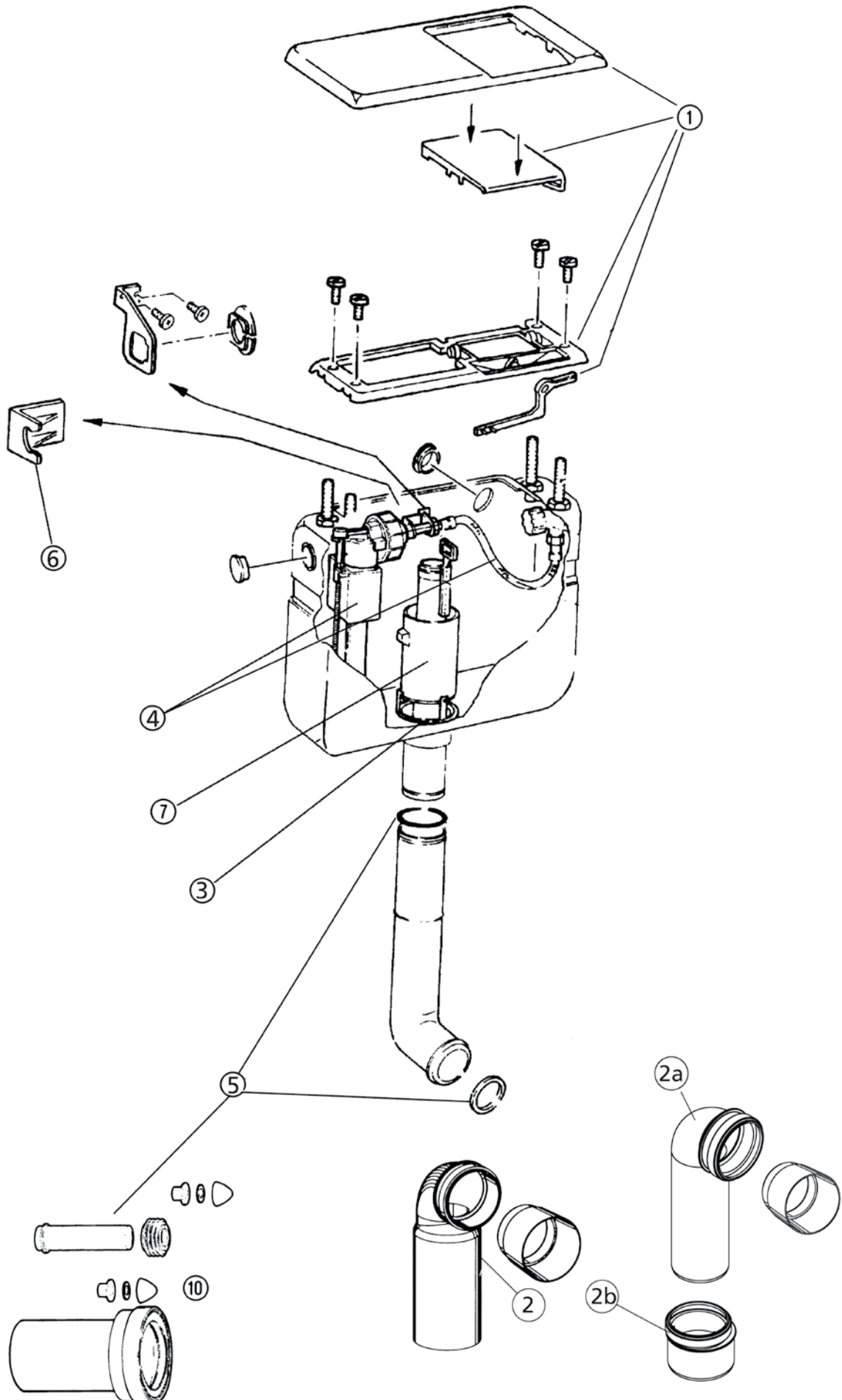
Schemat szczegółowy elementów do spłuczki TOP 6 / Accessories for concealed cistern TOP 6
