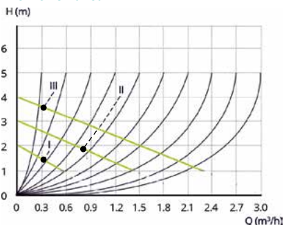
CI-PC 25/40-180
