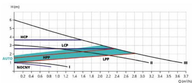
CI-PE-MERC 25/60/130, CI-PE-MERCURIO 25/60
