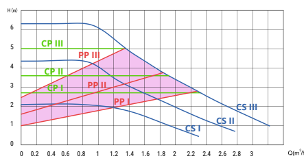
CI-TITANIO 25/60
