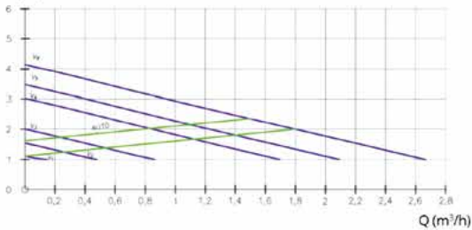
H(m) CI-HELIO 25/40-180
