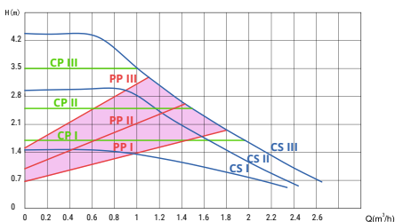
CI-TITANIO 25/40
