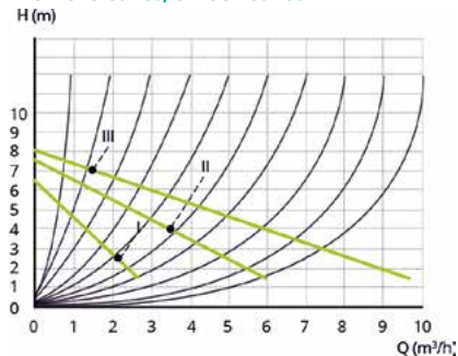
CI-PC 25/80-180, CI-PC 32/80-180
