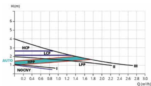
CI-PE-MERC 25/40
