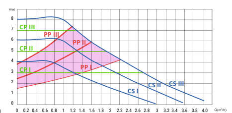
CI-TITANIO 25/80, CI-TITANIO 32/80
