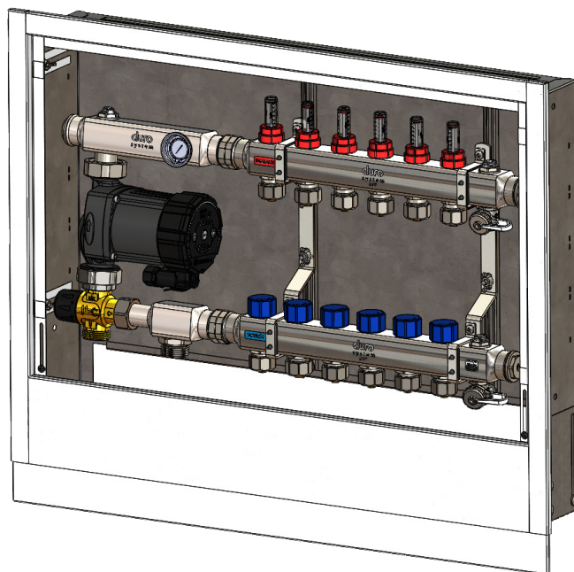
Rozdzielacz + układ mieszający
