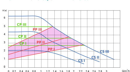
CI-TITANIO 25/60, CI-TITANIO 15/60
