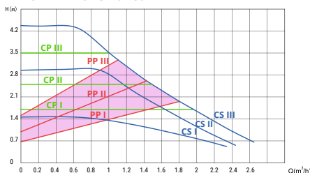
CI-TITANIO 25/40-180
