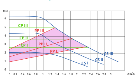
CI-TITANIO 25/60, CI-TITANIO 15/60
