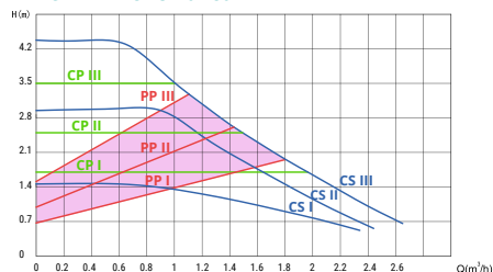
CI-TITANIO 25/40-180
