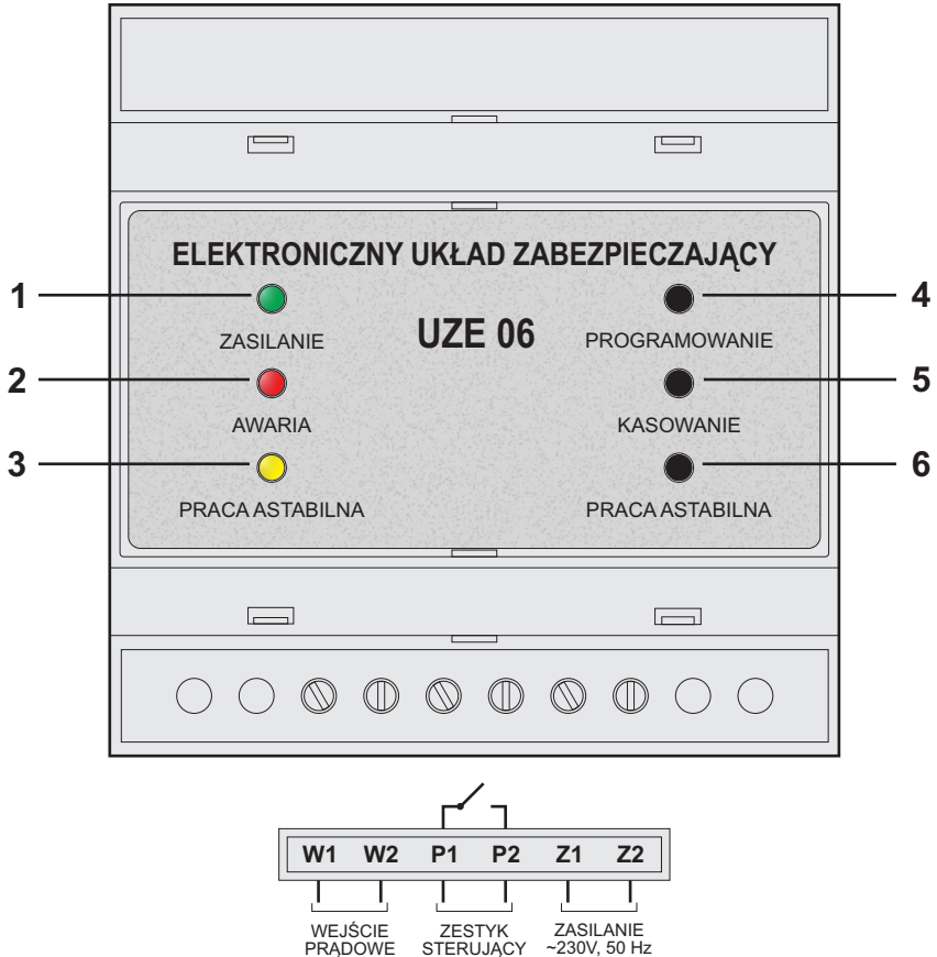
Rys. 1 Budowa układu
