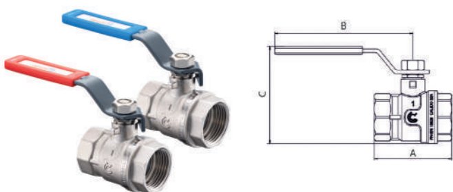
ZAWÓR GW/GW, DŹWIGNIA
