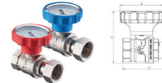
ZAWÓR KULOWY GW/GW Z RUCHOMĄ NAKRĘTKĄ, POKRĘTLEM I TERMOMETREM
