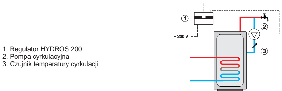
Rys. 3 Przykładowe podłączenie regulatora do instalacji ciepłej wody użytkowej z pompą cyrkulacyjną.
