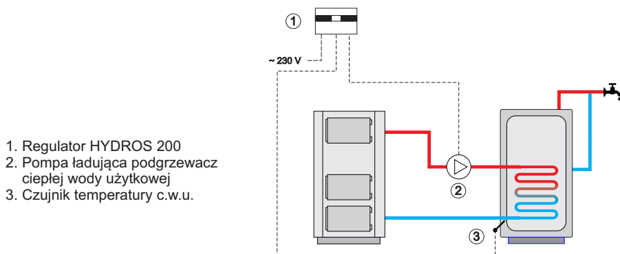
Rys. 2 Przykładowe podłączenie regulatora do instalacji z pompą ładującą podgrzewacz ciepłej wody użytkowej.
