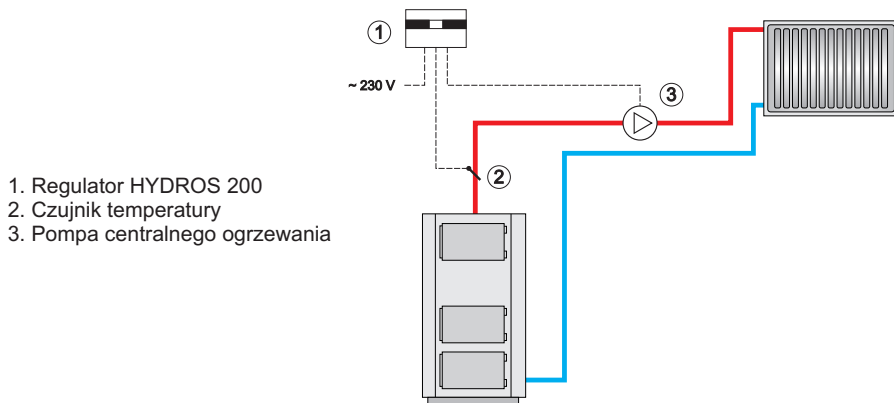
Rys. 1 Przykładowy schemat instalacji grzewczej ze sterownikiem HYDROS 200.
